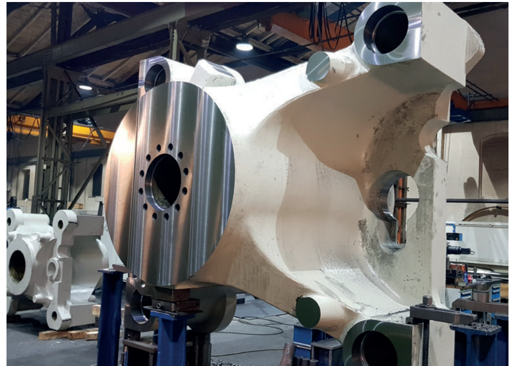
Presszylinder einer Kalksandsteinpresse
